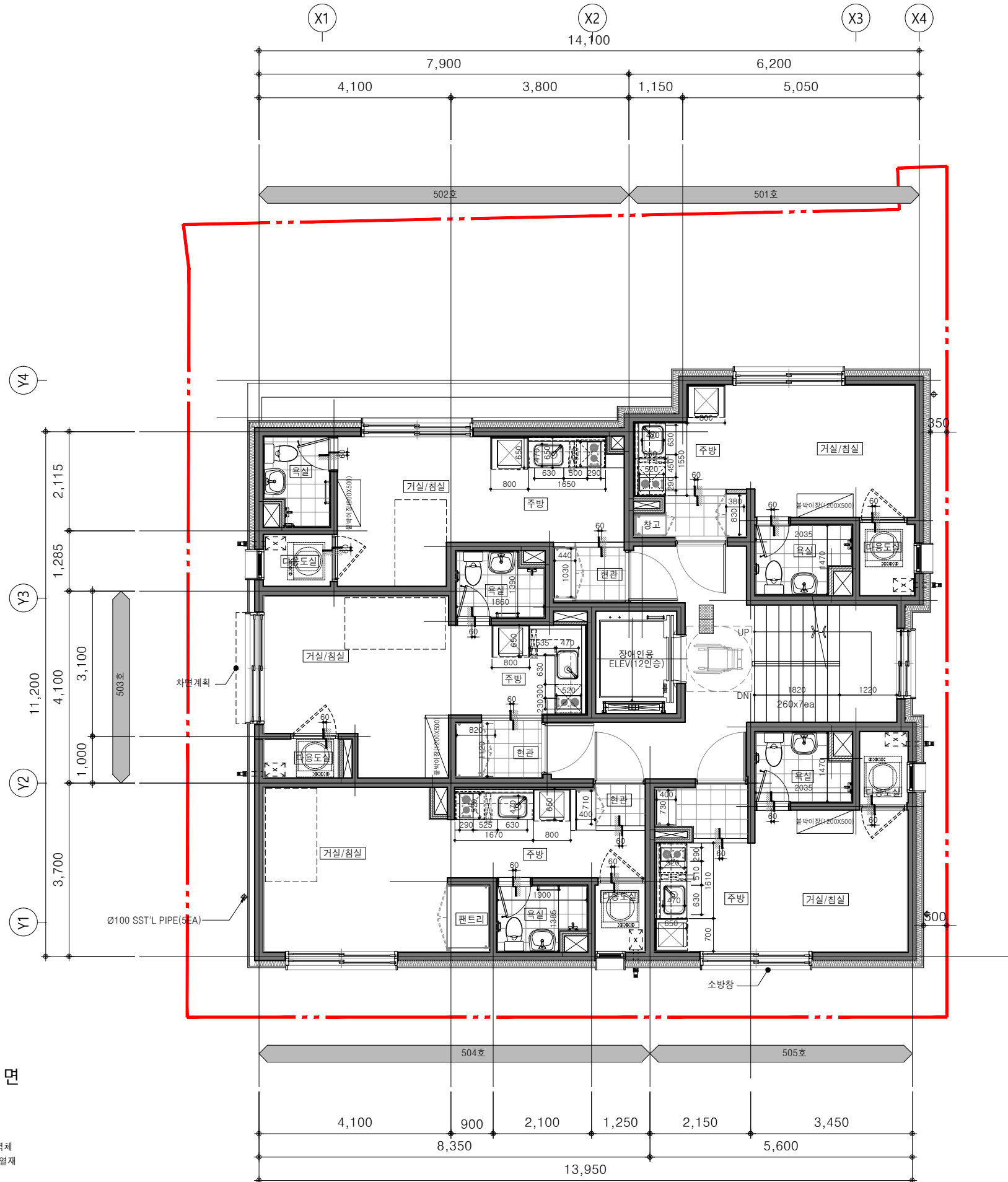
1 A 5층 평면도 SCALE : A3=1/100
