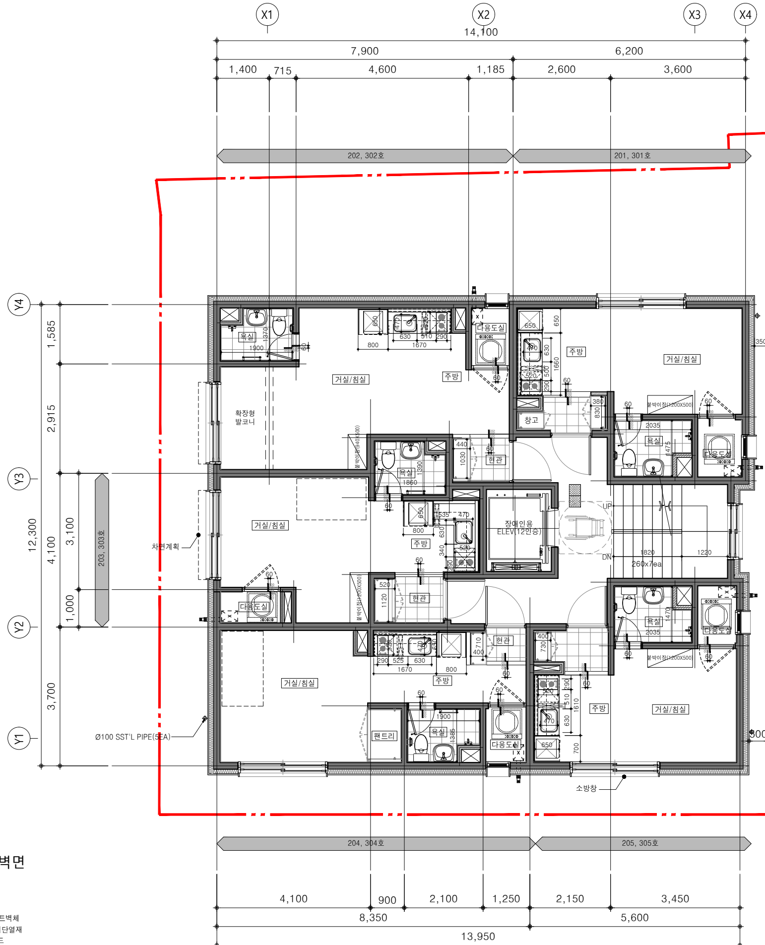
2~3층 평면도 SCALE : A3=1/100
