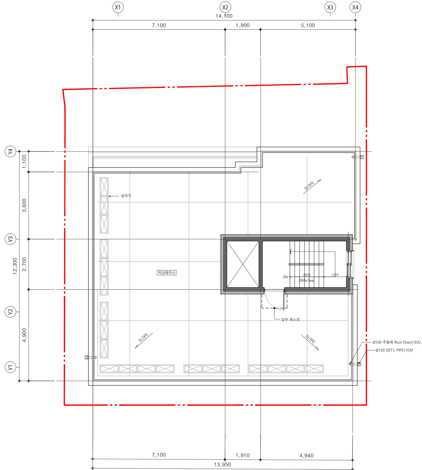
지붕층 평면도 SCALE : A3=1/100
