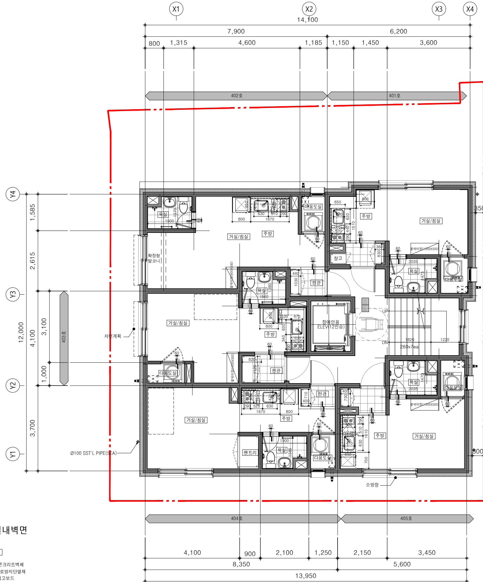
4층 평면도 SCALE : A3=1/100
